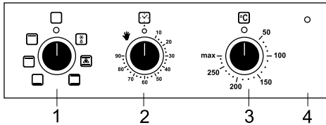
Рис. 1. Панель управления
