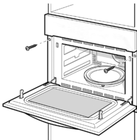
Крепление духового шкафа к мебели.
