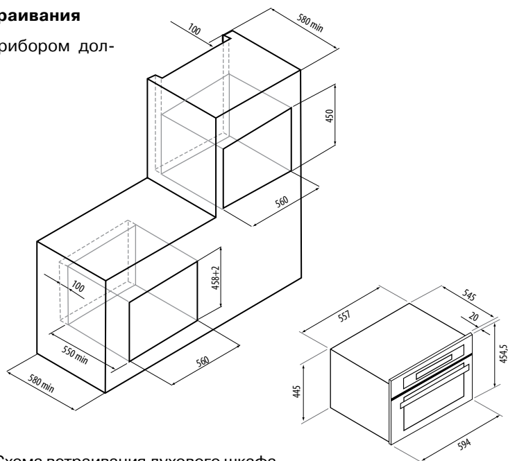
Схема встраивания духового шкафа.
