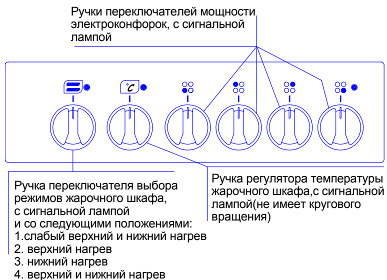
Рисунок 3 – Передняя панель плиты ЭП 401СТ
