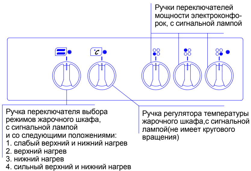
Рисунок 4 – Передняя панель плиты ЭП 301СТ
