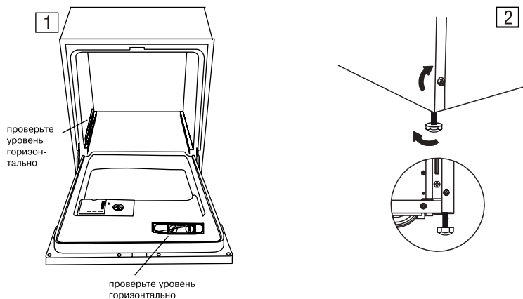
Рис. 8. Регулирование горизонтального положения машины.
