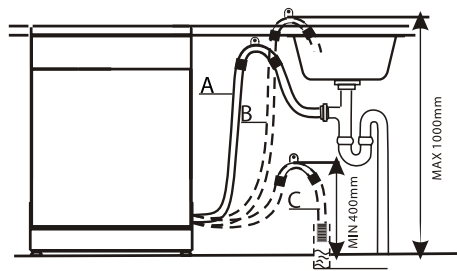
Рис.6. Подсоединение сливного шланга.
