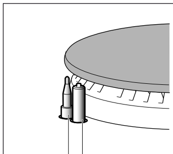
термопара | свеча
