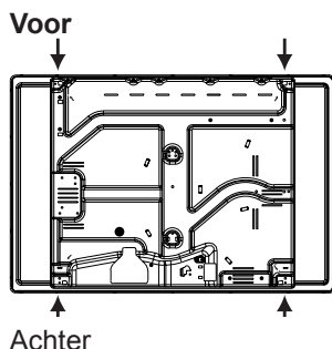
Stand haak voor keukenblad H=30mm
