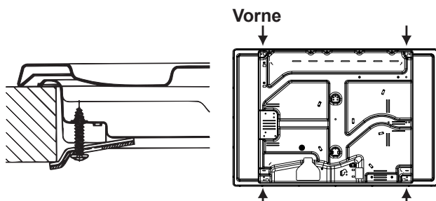
Position der Haken für Arbeitsplatten H=40mm
