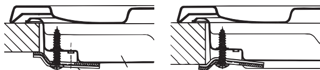
Position der Haken für Arbeitsplatten H=20mm
