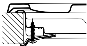
Монтаж крюка для опорных брусков H=40 мм
