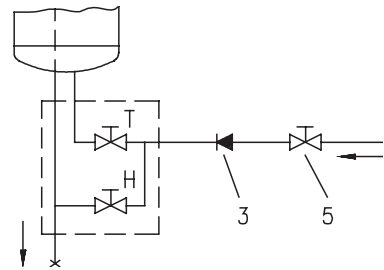
Odprti (netlačni) sistem
