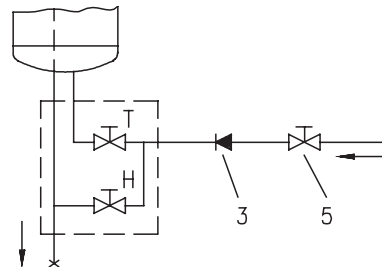
Système ouvert (à non-pression)
