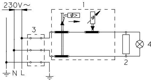
Das Schaltungsschema des Elektroanschlusse
