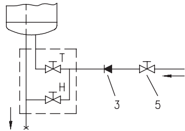
Das Durchflußsystem
