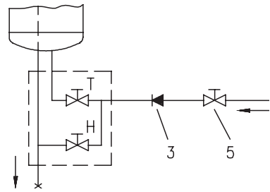
System otwarty (nieciśnieniowy)
