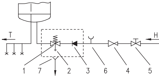
Zaprti (tlačni) sistem
