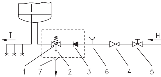
Sistemi (me shtypje) i mbyllur
