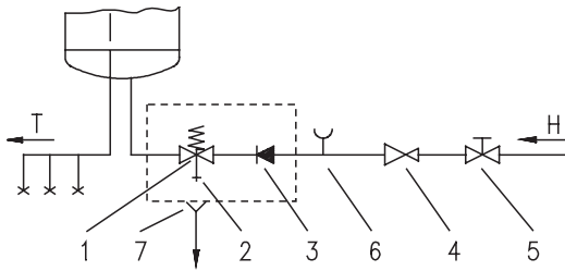
Système fermé (à pression)
